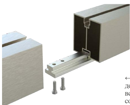
Профильное соединение P1 DAARTS SOL DS STRONG 70
